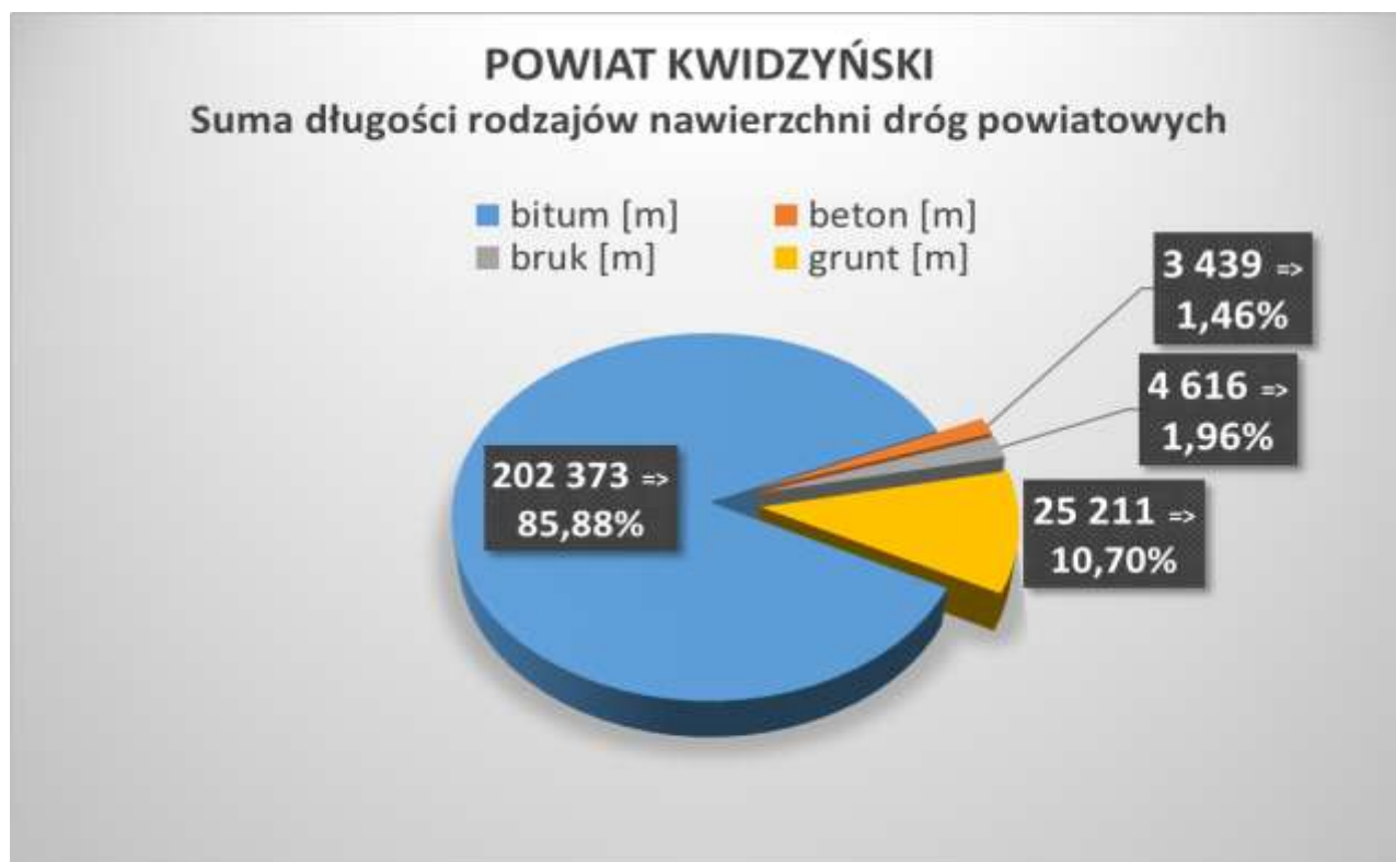
Wykres nr 10 – Suma długości rodzajów nawierzchni dróg powiatowych
